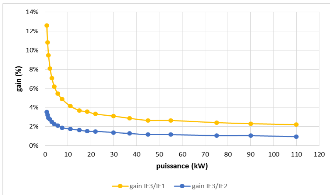
Figure 4 : Pourcentages des gains énergétiques obtenus en remplaçant des moteurs standards par des moteurs à haut rendement pour les moteurs électriques 4 pôles, 50 Hz
