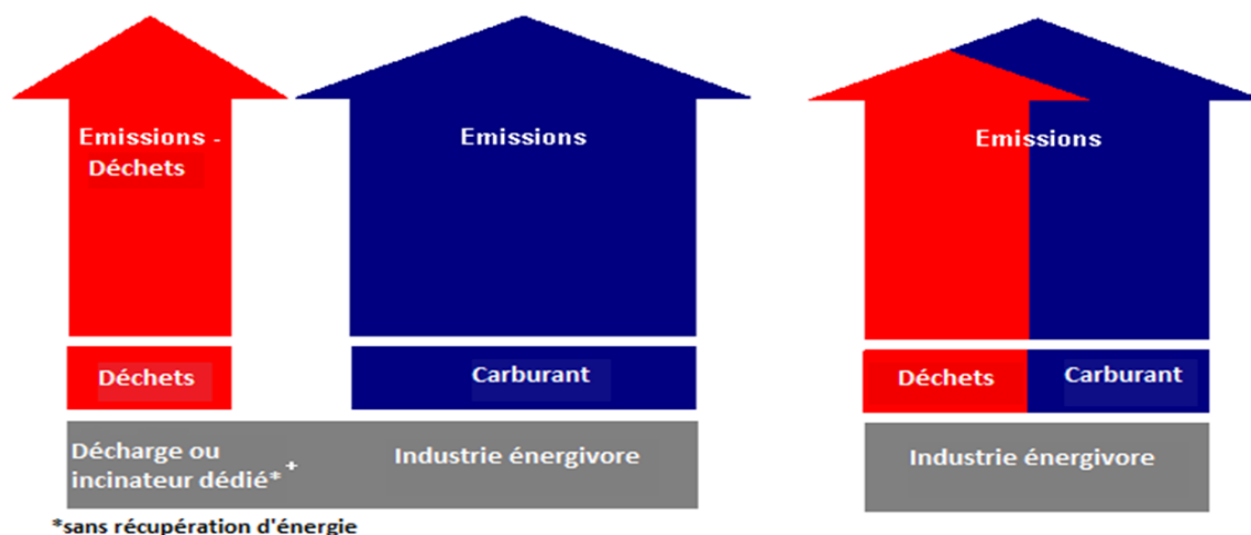
Figure 1: Schéma explicatif de la réduction des émissions de GES grâce au co-processing
