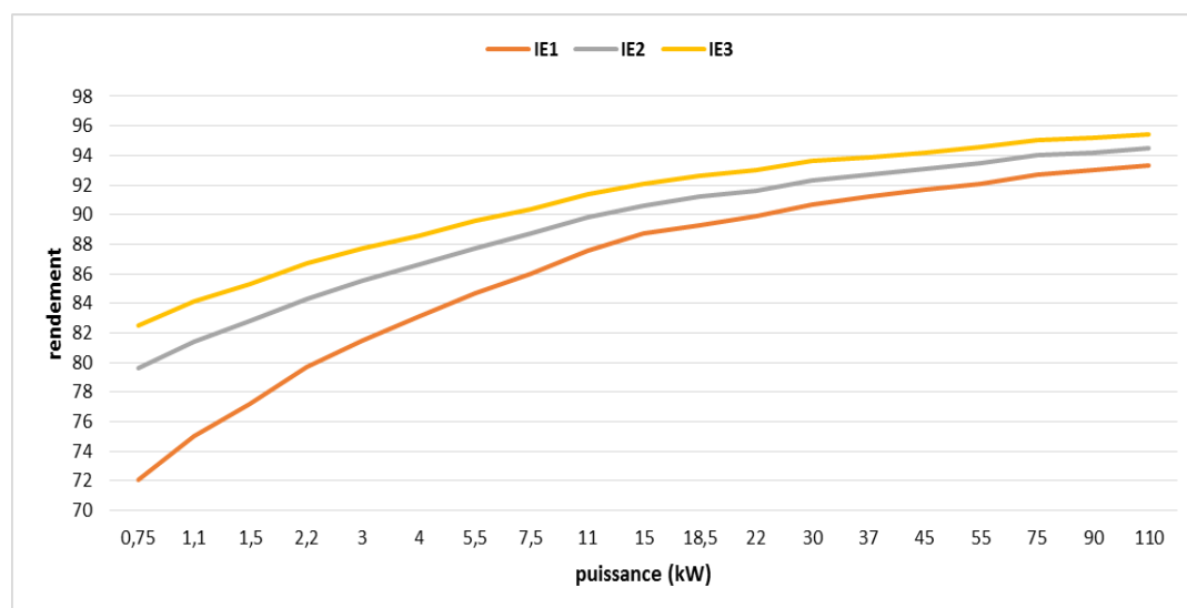
Figure 3 : Comparaison des valeurs limites des rendements IE1, IE2 et IE3 pour les moteurs électriques 4 pôles, 50 Hz
