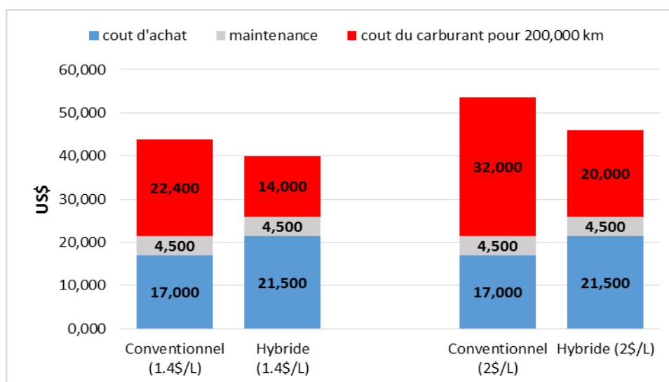
Figure 5 : Comparaison des coûts sur la durée de vie d'un véhicule classique et hybride
