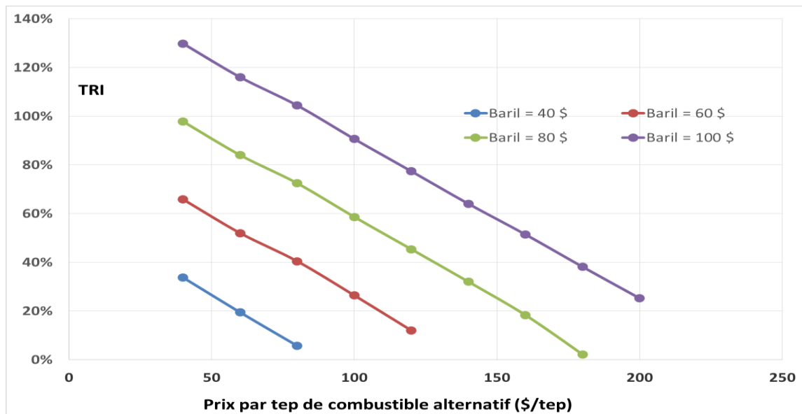
Figure 2 : TRI en fonction du prix de baril de pétrole et du prix du combustible alternatif utilisé dans la cimenterie
